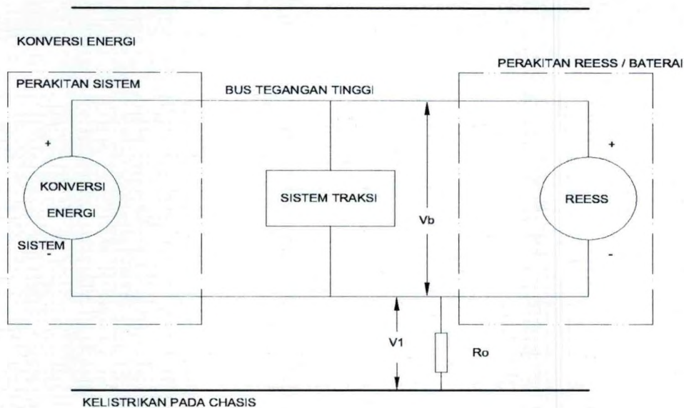
Gambar 2 Pengukuran V1'
