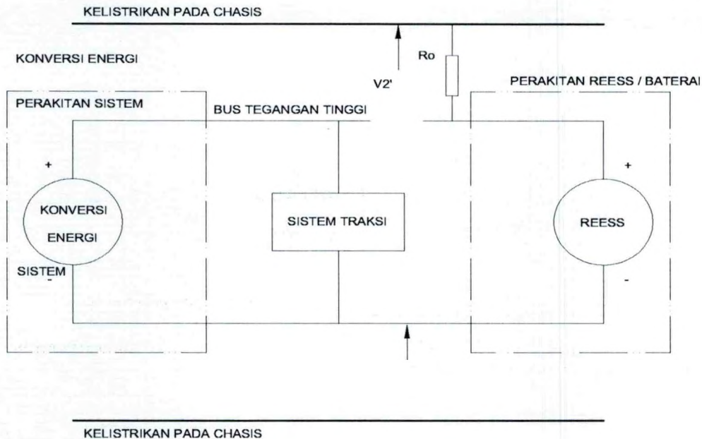
Gambar 3 Pengukuran V_2'
