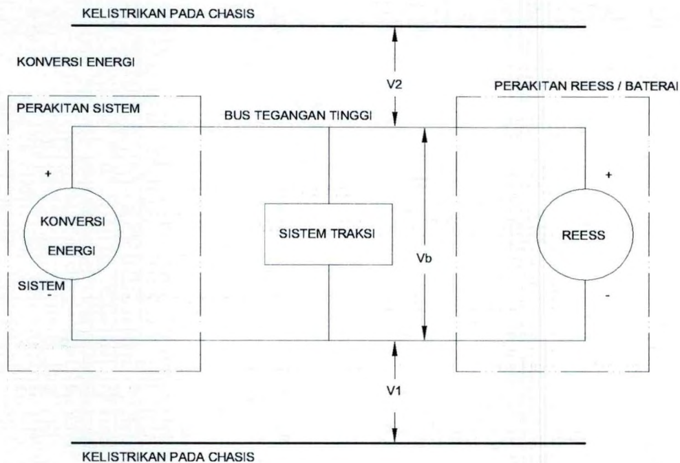
Gambar 1 Pengukuran Vb, V1, V2
