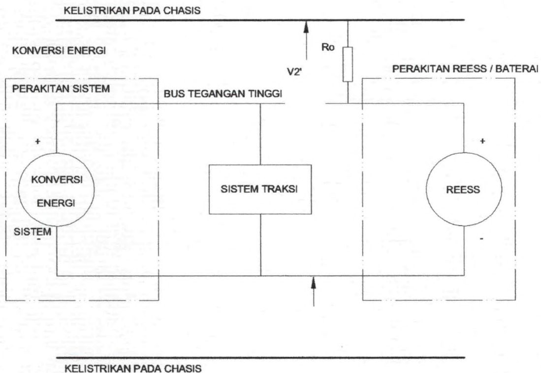
Gambar 3 Pengukuran V_2'
