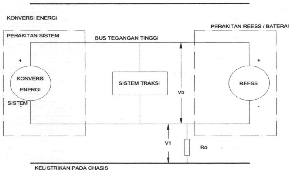
Gambar 2 Pengukuran V_1'
